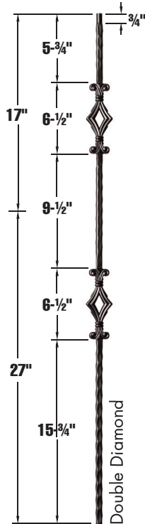
9041HF-_-44 10 pcs per box 490 pcs per skid
